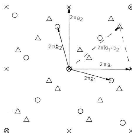
Abb. 1. Schnitt durch zwei reziproke Gitter; \times , \circ Punkte des reziproken Gitters von a, b; \Delta Doppelbeugungsreflexe; a_1, a_2 bzw. b_1, b_2 sind die Basisvektoren der reziproken Gitter von a bzw. b; es sind nicht alle möglichen Doppelbeugungsreflexe eingetragen.
